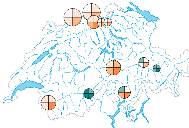
Veränderung der Jahresproduktion (GWh/Jahr)
