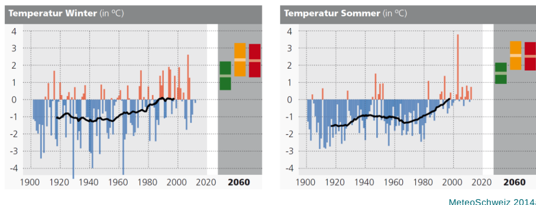
Figur 4: Bisher beobachtete sowie für 2060 projizierte Abweichung der Durchschnittstemperatur (in °C) gegenüber dem Mittel der Periode 1981-2010 (Projektion 2060 abhängig vom Emissionsszenario, s. Figur 3). Links: Winter / Rechts: Sommer Dicke Linie: 30-jähriges laufendes Mittel, rote/blau Säulen: Jahreswerte. Für 2060 werden jeweils die Bandbreiten der möglichen Änderungen sowie die mittlere Schätzung (heller Balken) gezeigt.
