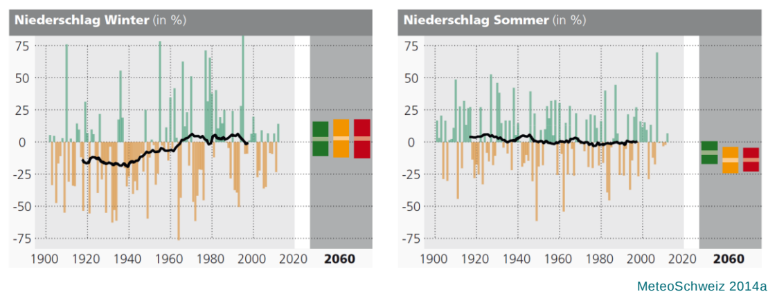
Figur 5: Bisher beobachtete sowie für 2060 projizierte Abweichung des Niederschlags (in %) gegenüber dem Mittel der Periode 1981-2010 (Projektion 2060 abhängig vom Emissionsszenario, s. Figur 3). Links: Winter / Rechts: Sommer Dicke Linie: 30-jähriges laufendes Mittel, gelbe/grüne Säulen: Jahreswerte. Für 2060 werden jeweils die Bandbreiten der möglichen Änderungen sowie die mittlere Schätzung (heller Balken) gezeigt.
