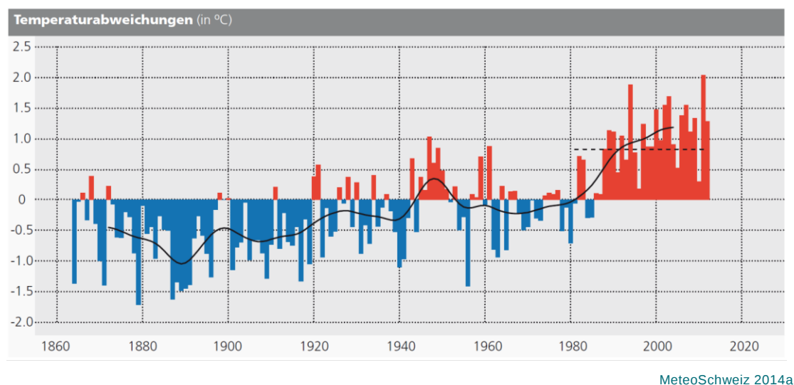
Figur 2: Dargestellt in rot und blau ist die jährliche Abweichung der Temperatur von der mittleren Temperatur der Periode 1961 bis 1990. Die schwarze Kurve zeigt den geglätteten Verlauf und die gestrichelte Linie das Niveau der mittleren Temperatur von 1981 bis 2010.
