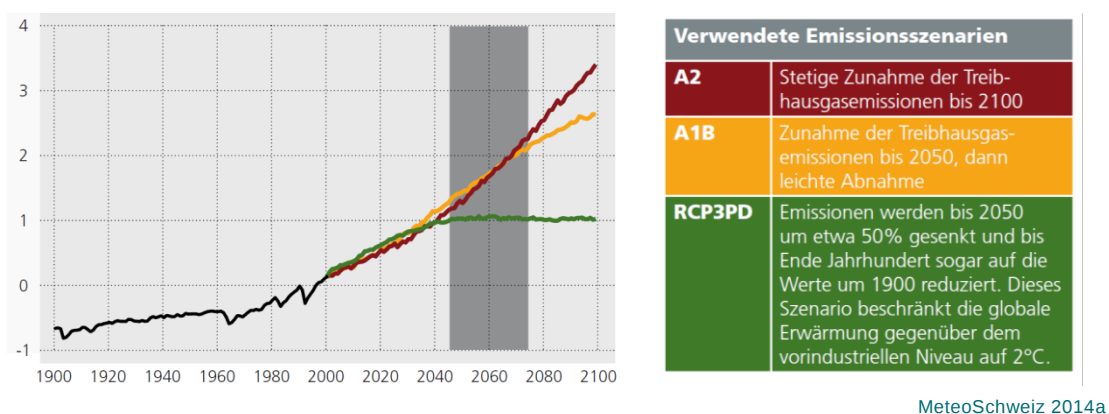
Figur 3: Links: Beobachtete und projizierte Abweichung der globalen Temperatur von der mittleren Temperatur der Periode 1981 bis 2010 in °C. Rechts: Szenarien der globalen Treibhausgasemissionen.
