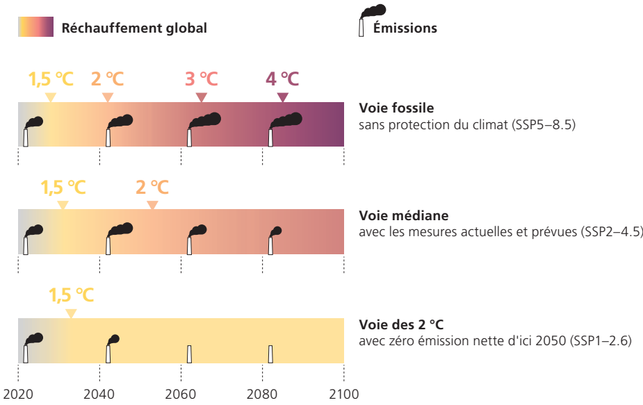
Estimation de l'année où un certain niveau de réchauffement climatique sera atteint
