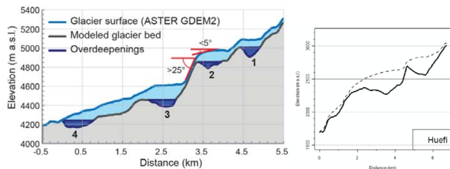
Abbildung 7: Längsprofil eines Gletschers zur Illustration der möglichen Übertiefungen in dessen Bett und ein Längsprofil des Hufifirns.
